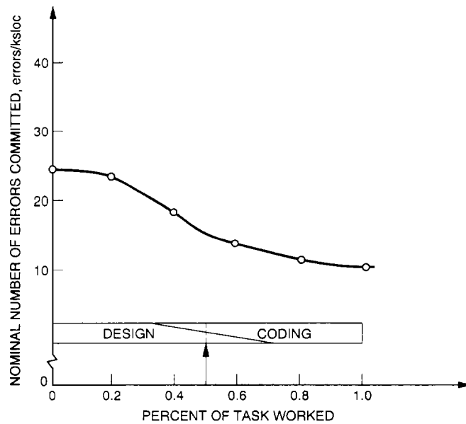
Fig. 6. Nominal errors generated per ksloc.
