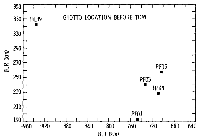
Fig. 8. Giotto B-Plane
