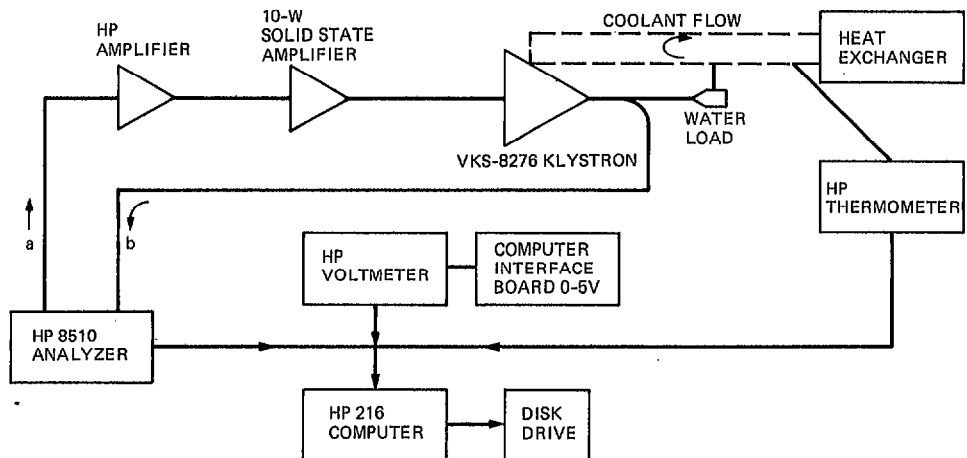
Fig. 1. Test setup
