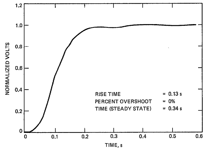
Fig. 23. Actual step response — azimuth axis loop, DSS 15
